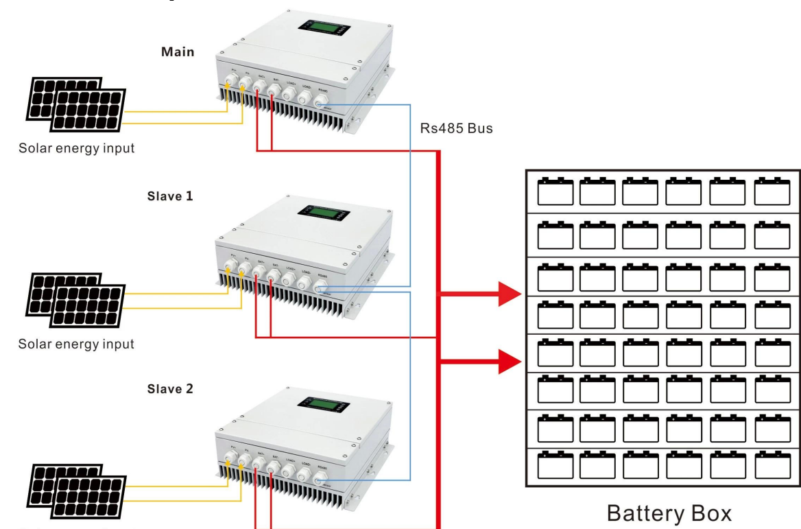
Schéma de connexion parallèle
