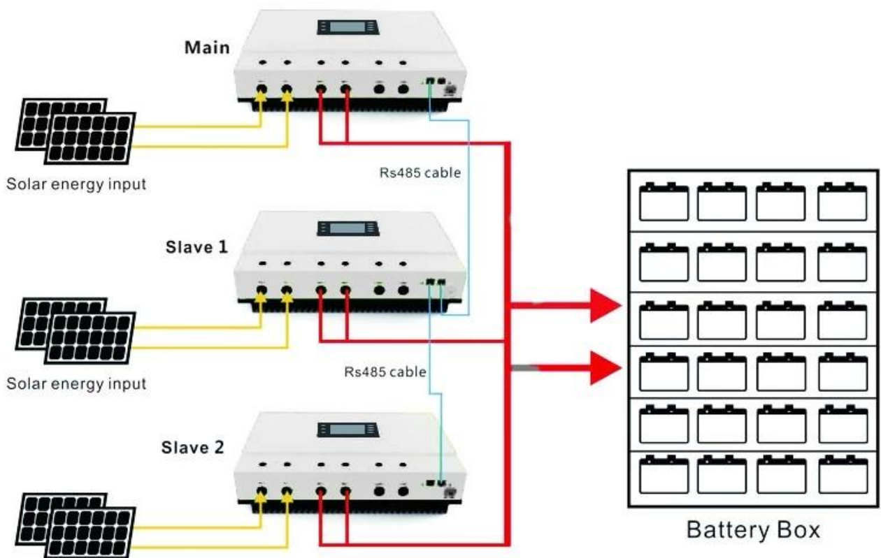
Diagrama de conexão paralelo
